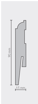
MP0901 90x15 mm SKIRTING 5905167674369 📏 2,42 m 📦 24,2 m 📦 847 m
