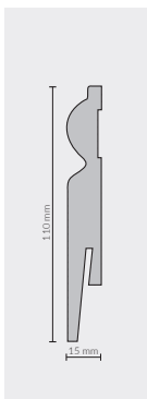
MP1101 110x15 mm SKIRTING 5905167674420 📏 2,42 m 📦 24,2 m 📦 847 m
